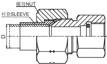
JIC外螺纹 74° 外锥 / 英管内螺纹表接头 JIC MALE 74° CONE / BSP PRESSURE GAUGE CONNECTOR
