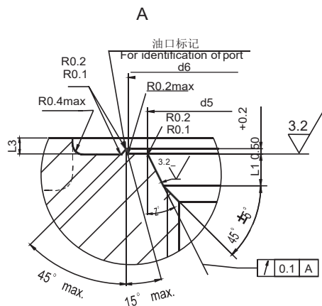
ISO 6149-1油口 ISO 6149-1 Port
