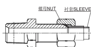
美制NPT外螺纹/ 美制 JIC外螺纹外锥过板接头 NPT MALE/JIC MALE 74° Cone Bulkhead
