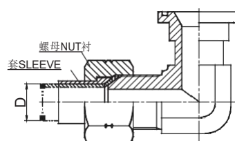
90° 弯美制JIC外螺纹74° 外锥 / 轻系列法兰ISO 6162-1 90° ELBOW JIC MALE 74° CONE / L-SERIES FLANGE ISO 6162-1
