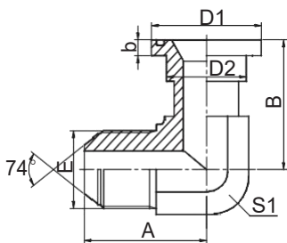
90° 弯美制JIC外螺纹74° 外锥 / 重系列法兰ISO 6162-2 1JFS9 90° ELBOW JIC MALE 74° CONE / S-SERIES FLANGE ISO 6162-2
