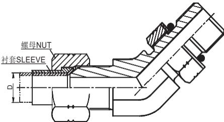
45° 弯JIC外螺纹74° 外锥 / SAE外螺纹带O形圈轻 系列ISO 11926-3 45° ELBOW JIC MALE 74° CONE / SAE O-RING BOSS L-SERIES ISO 11926-3
