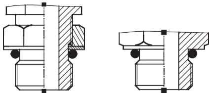
ISO 6149-2、ISO 6149-3柱端 ISO 6149-2、ISO 6149-3 stud end
