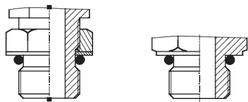
JIS B 2351 柱端 JIS B 2351 stud end
