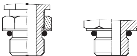
ISO 11926-2、ISO 11926-3美制螺纹柱端
