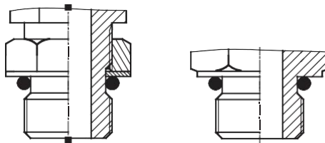
BS 5380柱端 BS 5380 stud end
